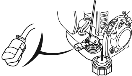
Рис. 18 Топливный фильтр
