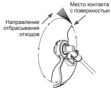
Рис. 14 Положение триммерной головки при удалении растительного покрова и обработке границы газона
