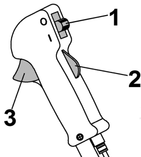
Рис. 2 Рукоятка управления
